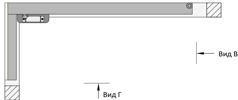
Вид сверху (в разрезе)
