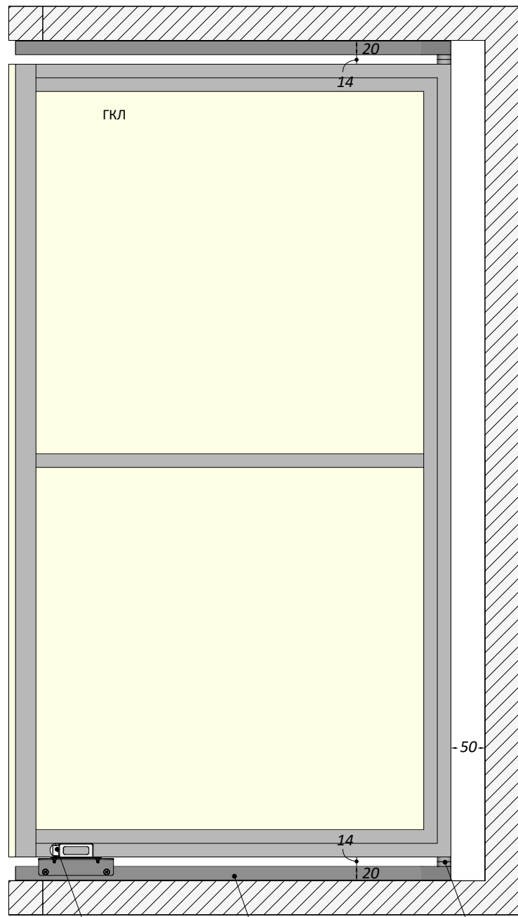
Вид сзади (Вид Г)
