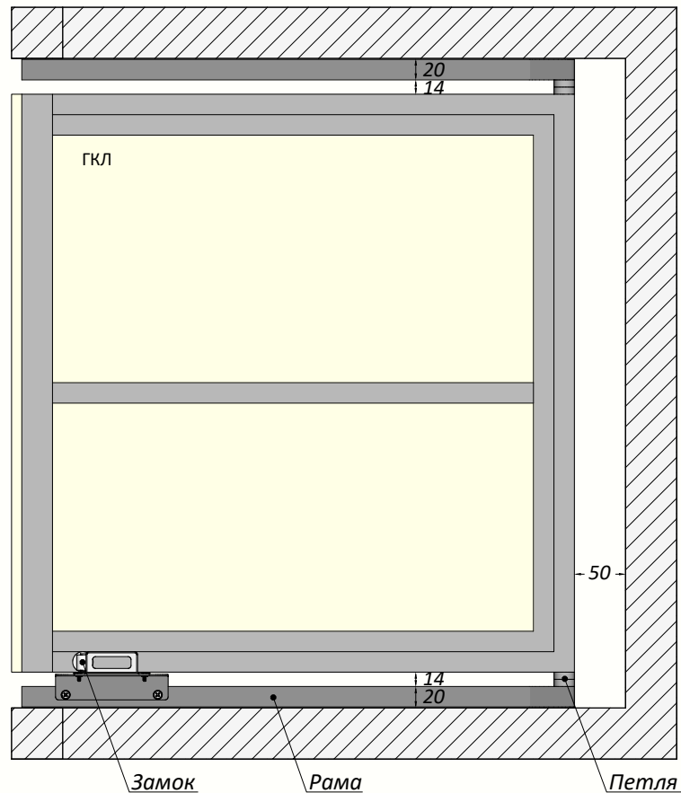
Вид сверху (в разрезе)
