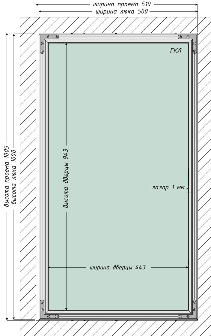
Вид спереди
