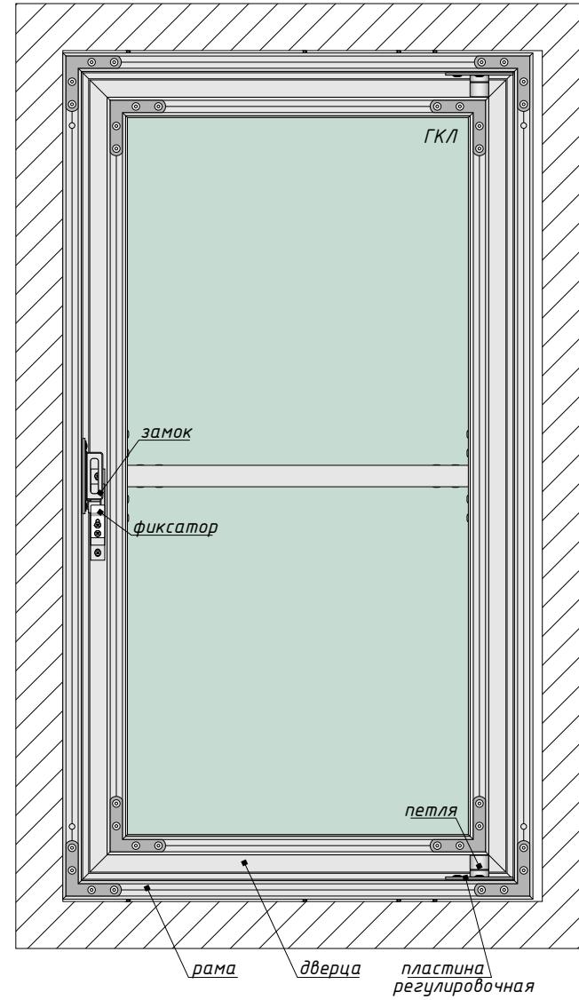
Вид сзади
